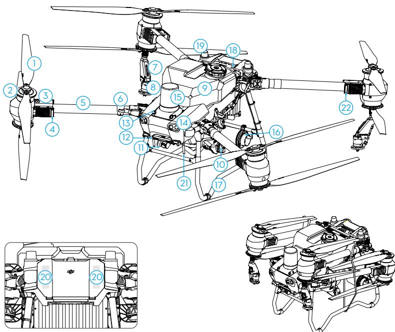
后视图
