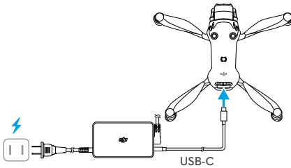
DJI Mavic 240W 電源アダプター
