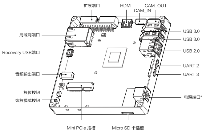
接口总览
