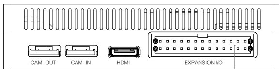
扩展口位置
