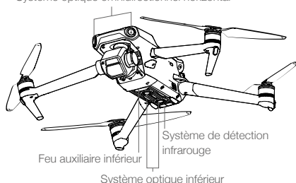
Système optique omnidirectionnel horizontal
