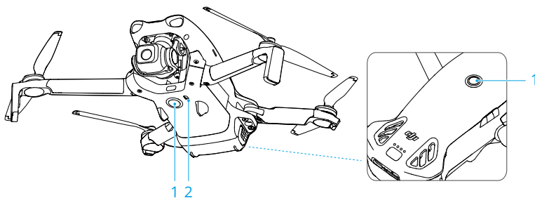
1. نظام الرؤية الأحادية متعددة الاتجاهات 2. نظام الاستشعار بالأشعة تحت الحمراء أسفل الطائرة
